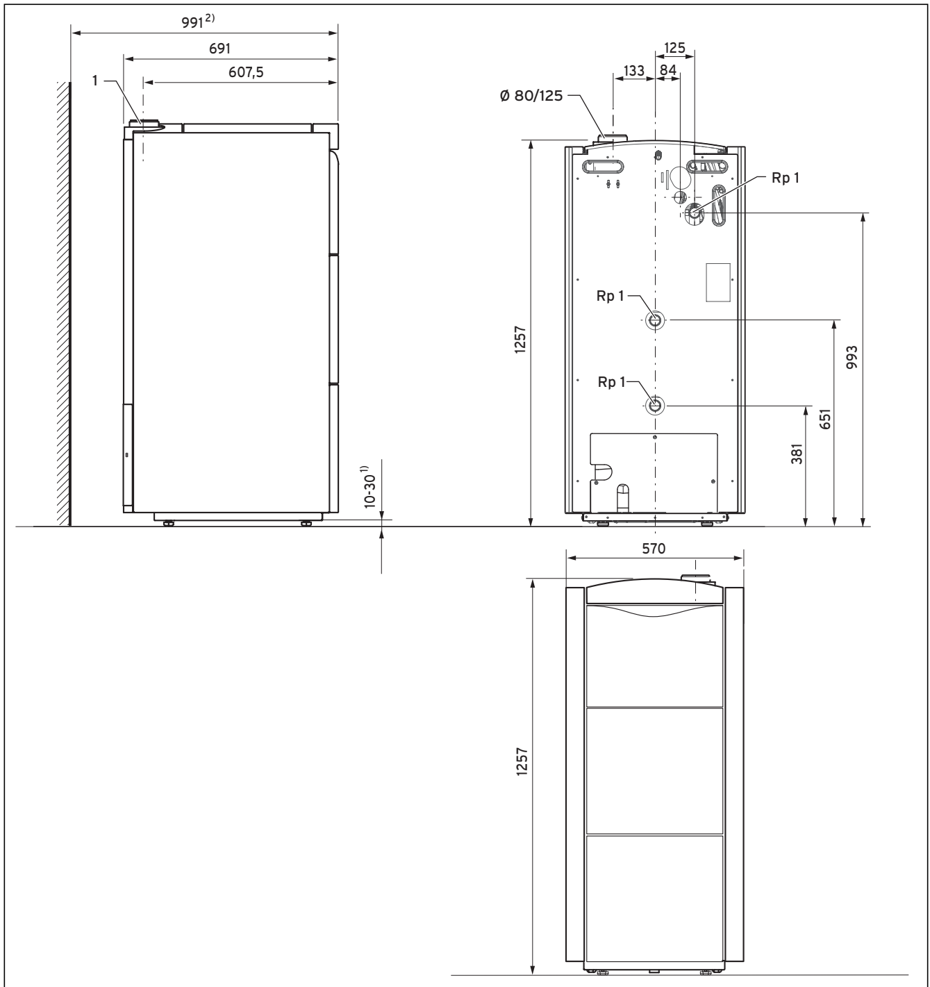
Мал. 4.2 Розміри
